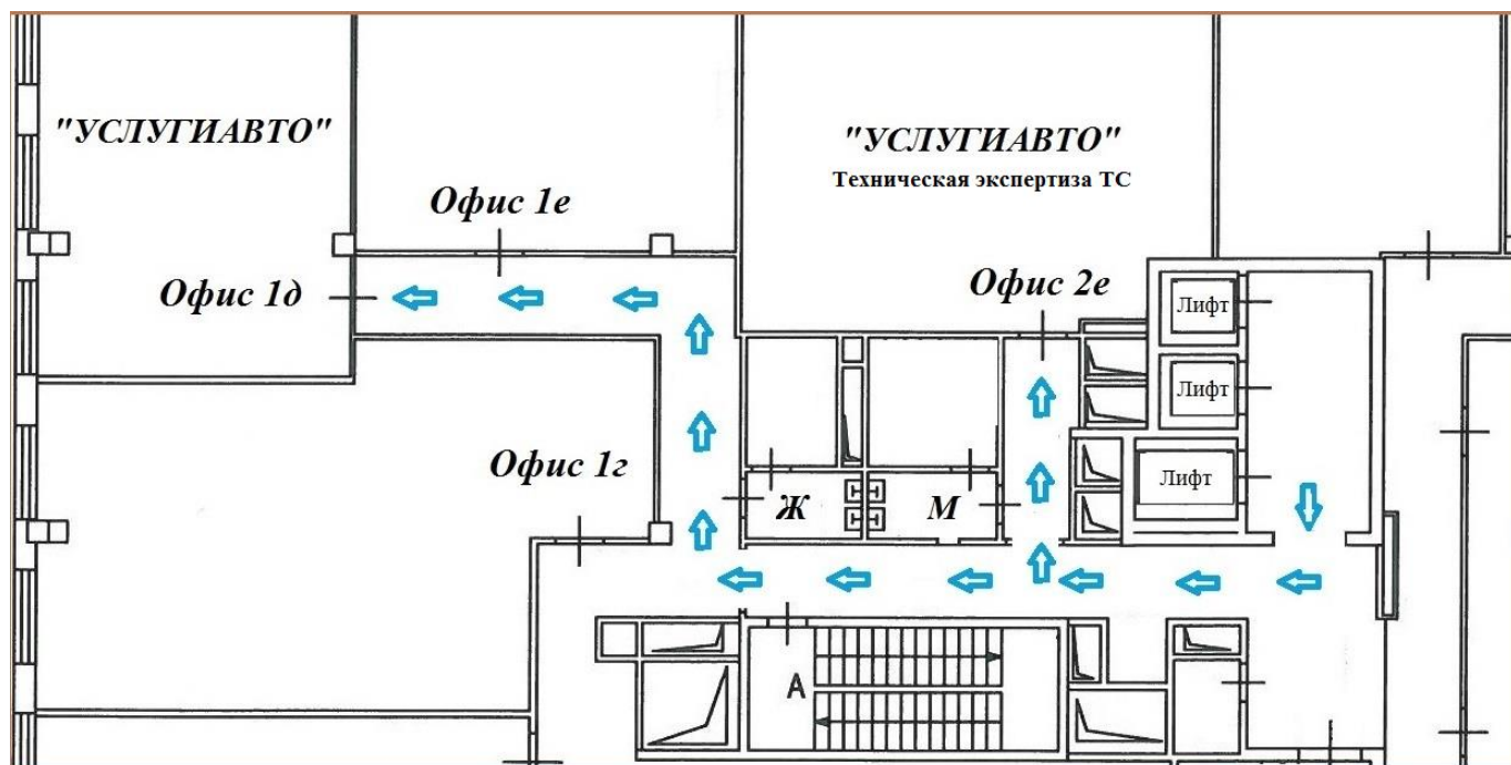
Схема (7 этаж)
